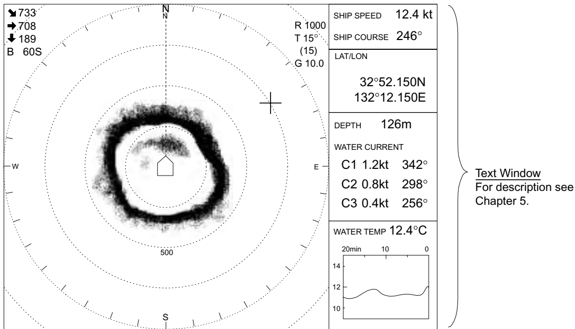
Sonar display
